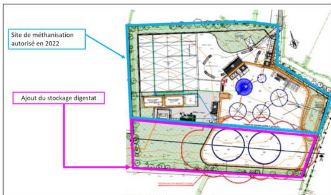
Figure 5 : Plan d'implantation du stockage
