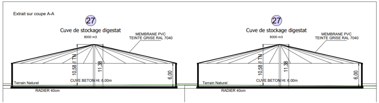
Figure 6 : Plan en coupe
